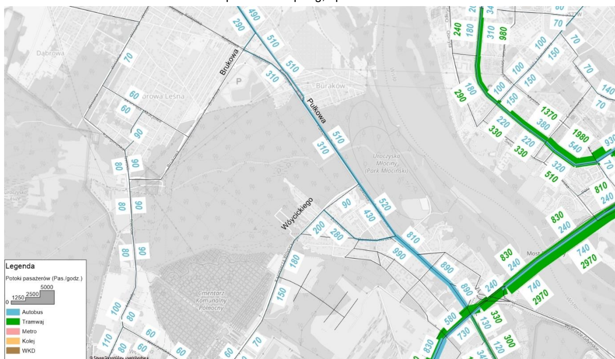
Rys. 6.9. Liczba pasażerów w transporcie zbiorowym w stanie istniejącym– rok 2018, godzina szczytu popołudniowego.
