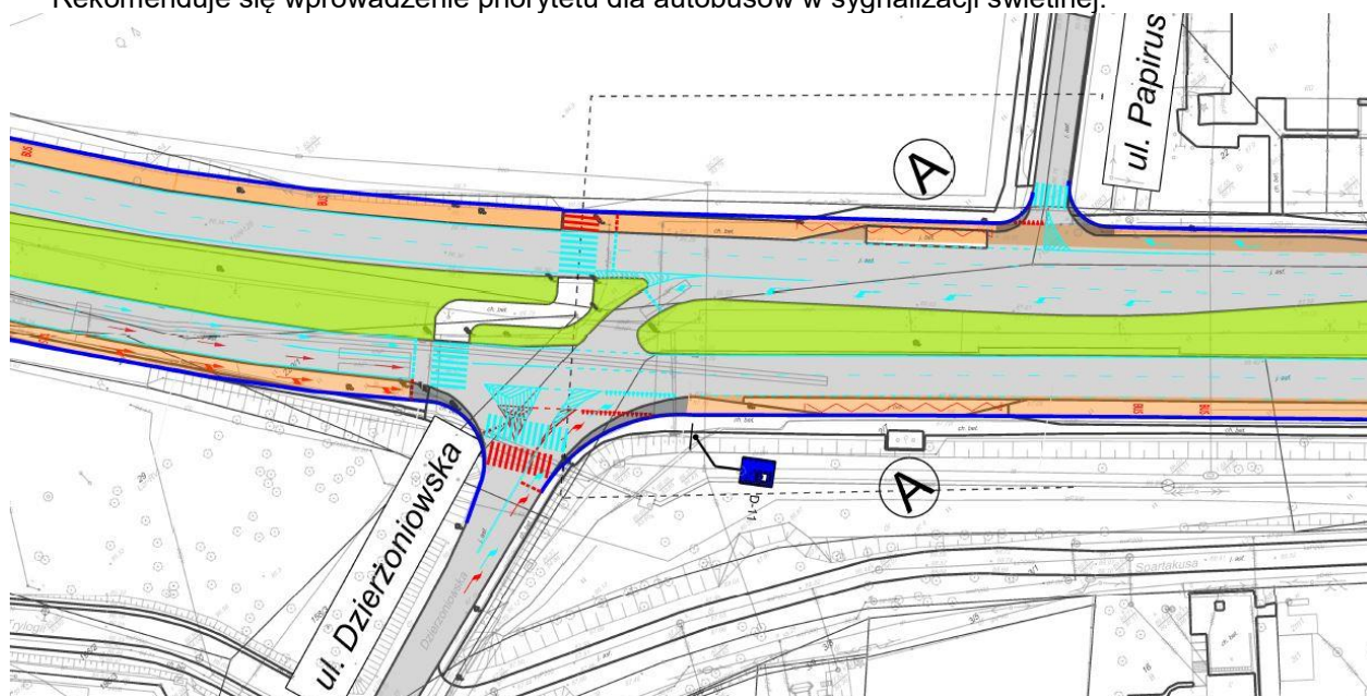
Rys. 5.19. Pas autobusowy w rejonie skrzyżowania ul. Pułkowej z ul. Dzierżoniowską – wariant 1b.
