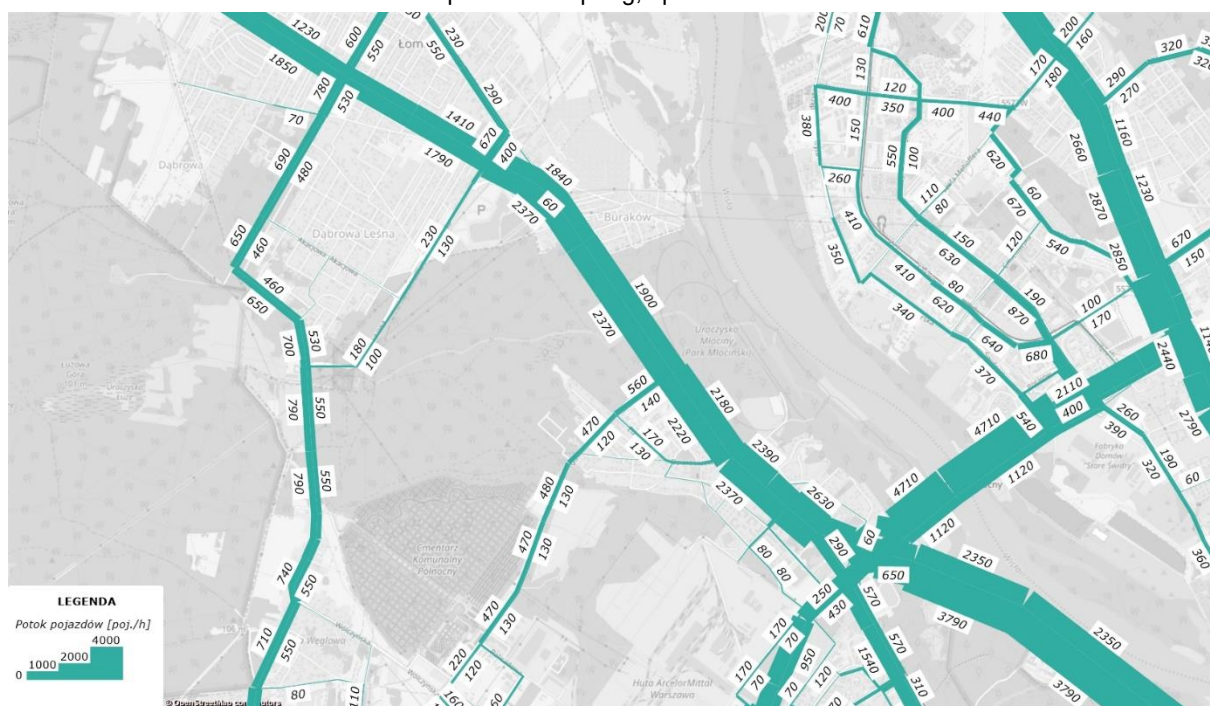
Rys. 6.22 Prognoza ruchu drogowego w szczycie porannym w roku 2020 - warianty inwestycyjne WA i WB źródło:openstreetmap.org, opracowanie własne
