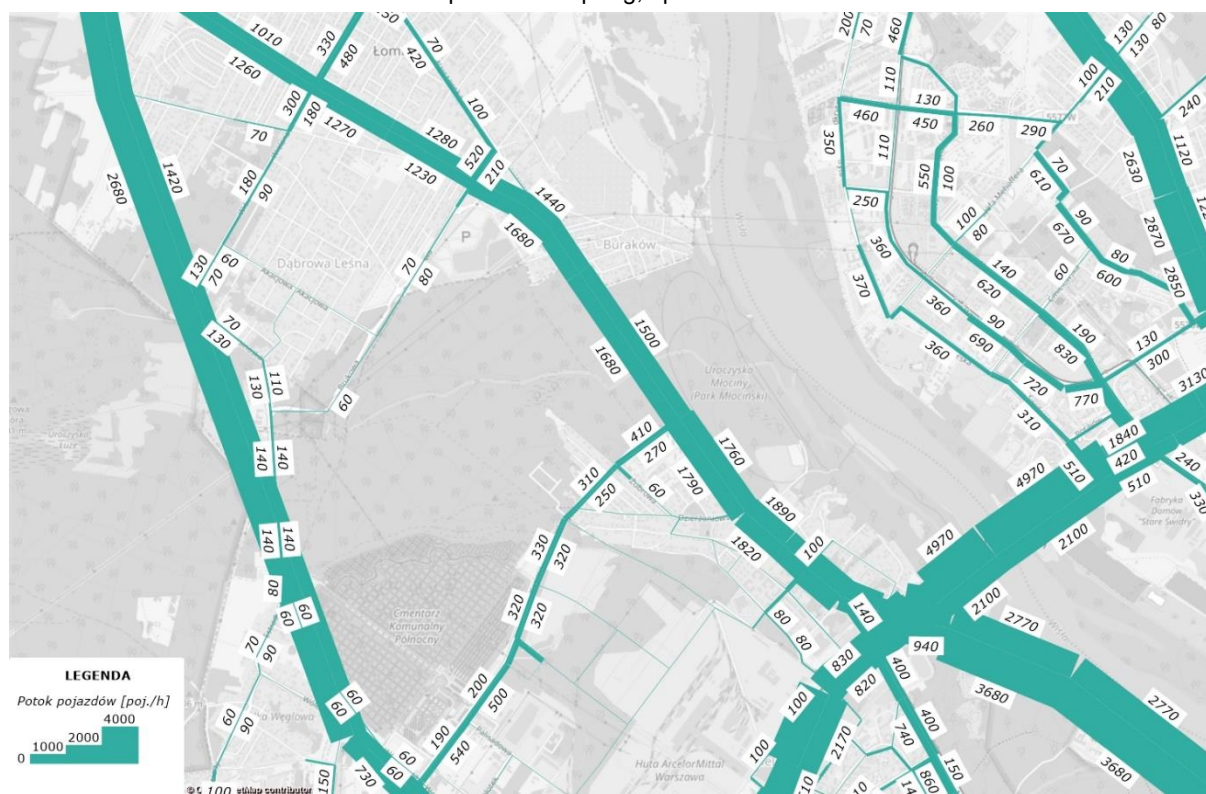
Rys. 6.30 Prognoza ruchu drogowego w szczycie porannym w roku 2025 - wariant bezinwestycyjny W0 źródło:openstreetmap.org, opracowanie własne
