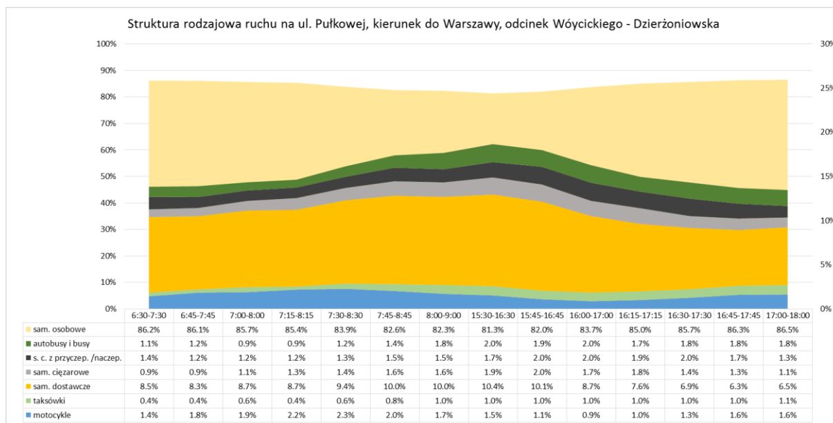
Rys. 4.20 Wyniki pomiarów ruchu, struktura rodzajowa ruchu na ul. Pułkowej, kierunek do Warszawy, odcinek Wóycickiego - Dzierżoniowska (źródło: opracowanie własne)
