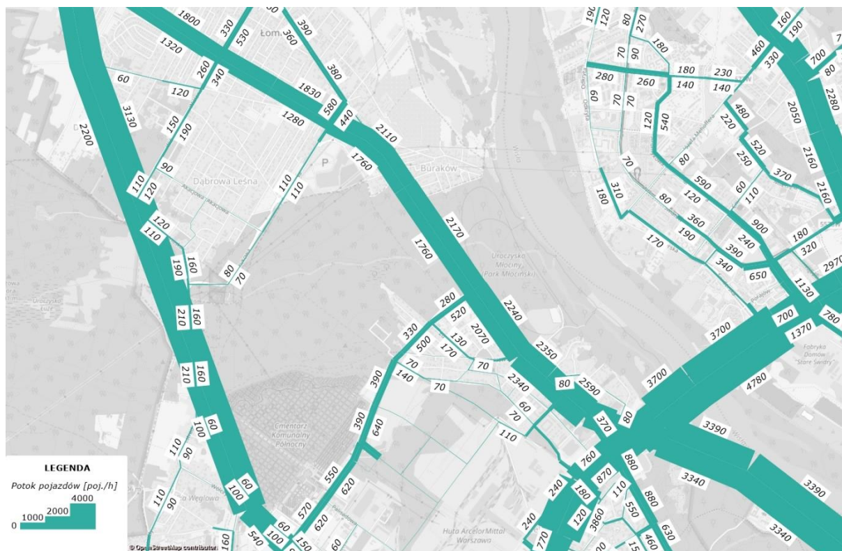
Rys. 6.45 Prognoza ruchu drogowego w szczycie popołudniowym w roku 2045 - warianty inwestycyjne WA i WB źródło: openstreetmap.org, opracowanie własne
