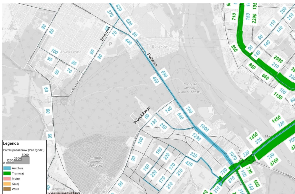
Rys. 6.43. Prognoza liczba pasażerów w szczycie popołudniowym w roku 2045 - wariant inwestycyjny WB źródło:openstreetmap.org, opracowanie własne
