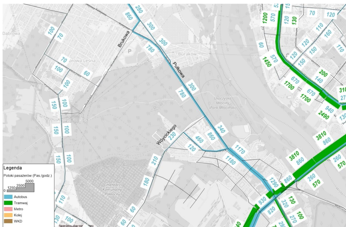
Rys. 6.19. Prognoza liczby pasażerów w szczycie porannym w roku 2020 – wariant bezinwestycyjny W0 źródło:openstreetmap.org, opracowanie własne
