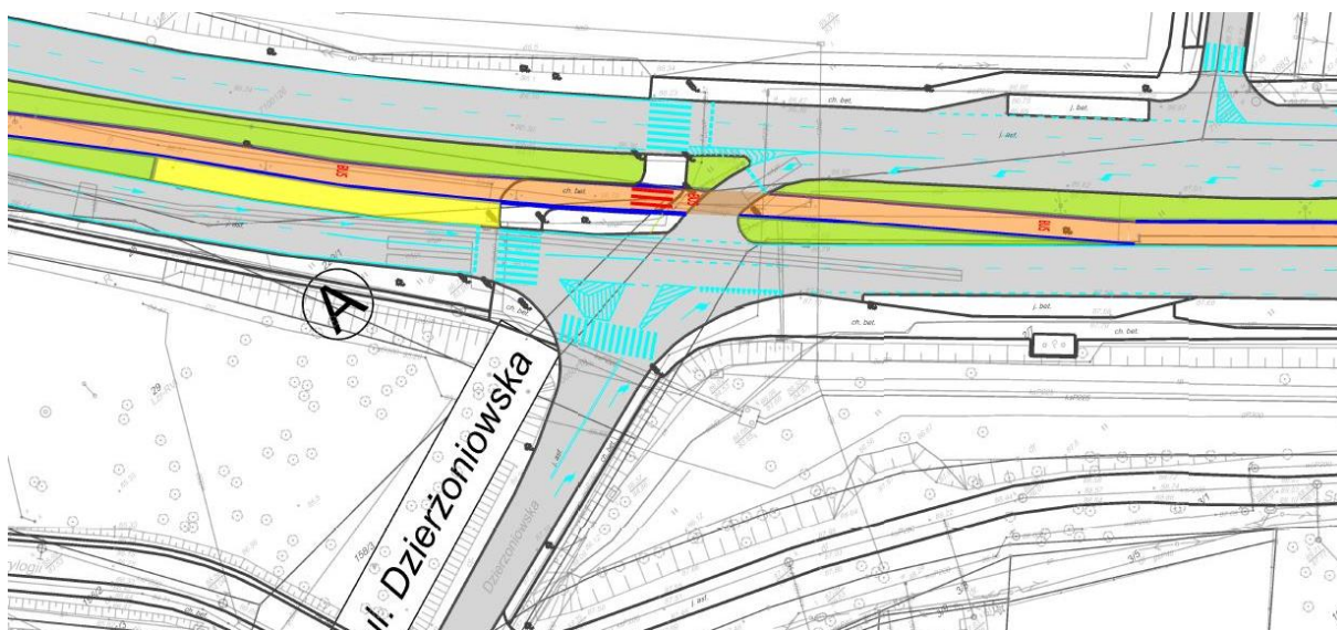
Rys. 5.31. Pas autobusowy, na skrzyżownaiu ul. Pułkowej z ul. Dzierżoniowską oraz lokalizacja platformy przystankowej dla przystanku „Dzierżoniowska” – wariant 2a.
