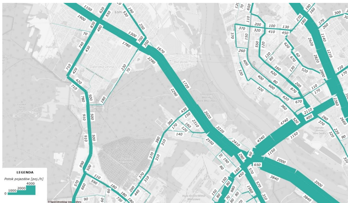
Rys. 6.6 Rozkład ruchu dla stanu istniejącego – rok 2018, godzina szczytu porannego.
