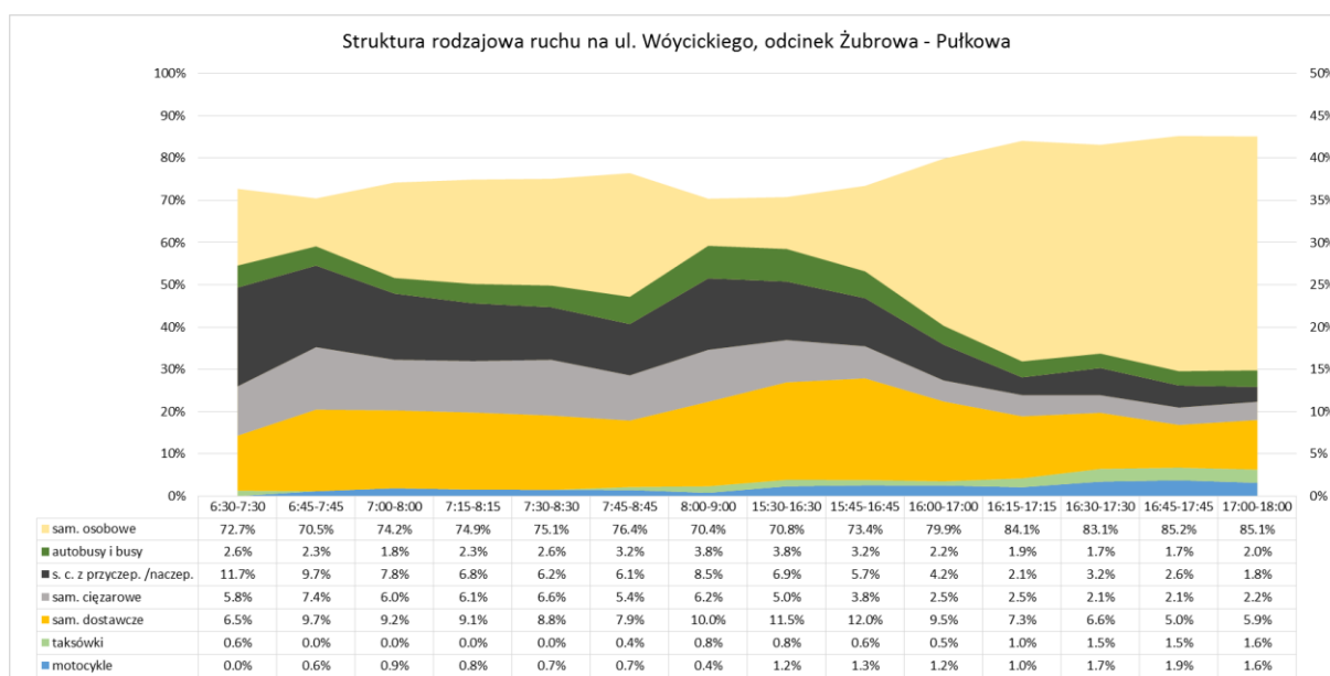
Rys. 4.22 Wyniki pomiarów ruchu, struktura rodzajowa ruchu na ul. Wóycickiego, odcinek Żubrowa - Pułkowa (źródło: opracowanie własne)
