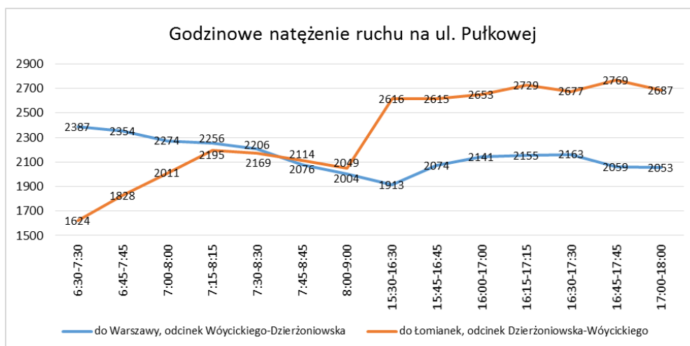
Rys. 4.16 Wyniki pomiarów ruchu na ul. Pułkowej pomiędzy ul. Wóycickiego i Dzierżonowską, interwały godzinowe, wszystkie pojazdy.
