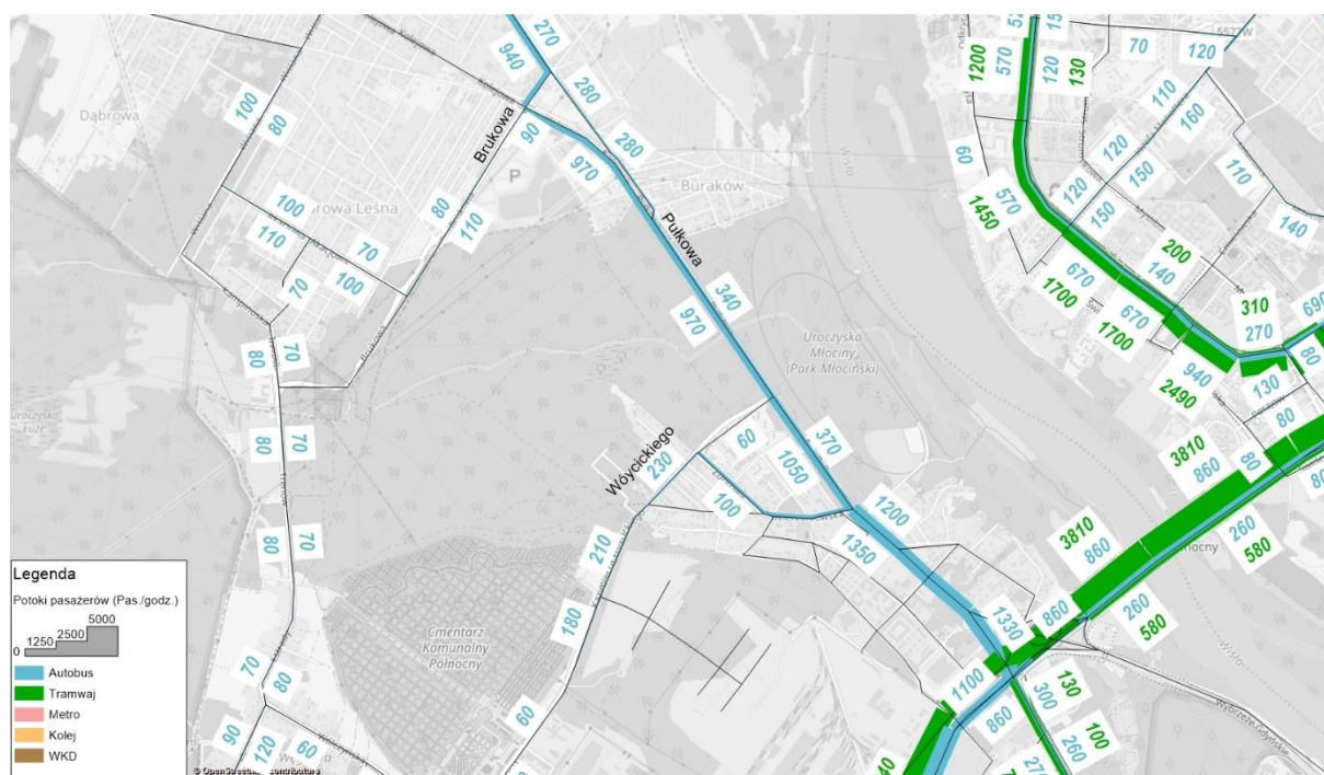
Rys. 6.20. Prognoza liczby pasażerów w szczycie porannym w roku 2020 - warianty inwestycyjne WA i WB źródło:openstreetmap.org, opracowanie własne
