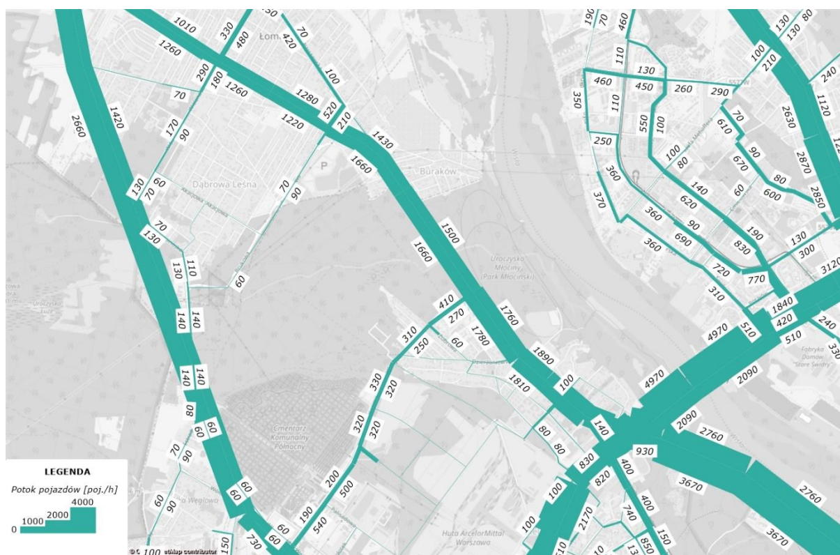
Rys. 6.31 Prognoza ruchu drogowego w szczycie porannym w roku 2025 - warianty inwestycyjne WA i WB źródło:openstreetmap.org, opracowanie własne
