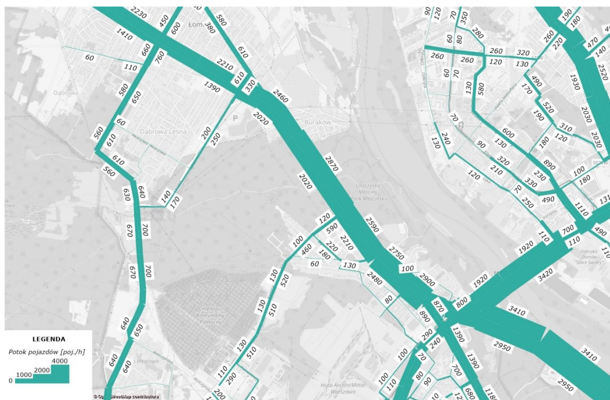
Rys. 6.26 Prognoza ruchu drogowego w szczycie popołudniowym w roku 2020 - wariant bezinwestycyjny W0 źródło:openstreetmap.org, opracowanie własne
