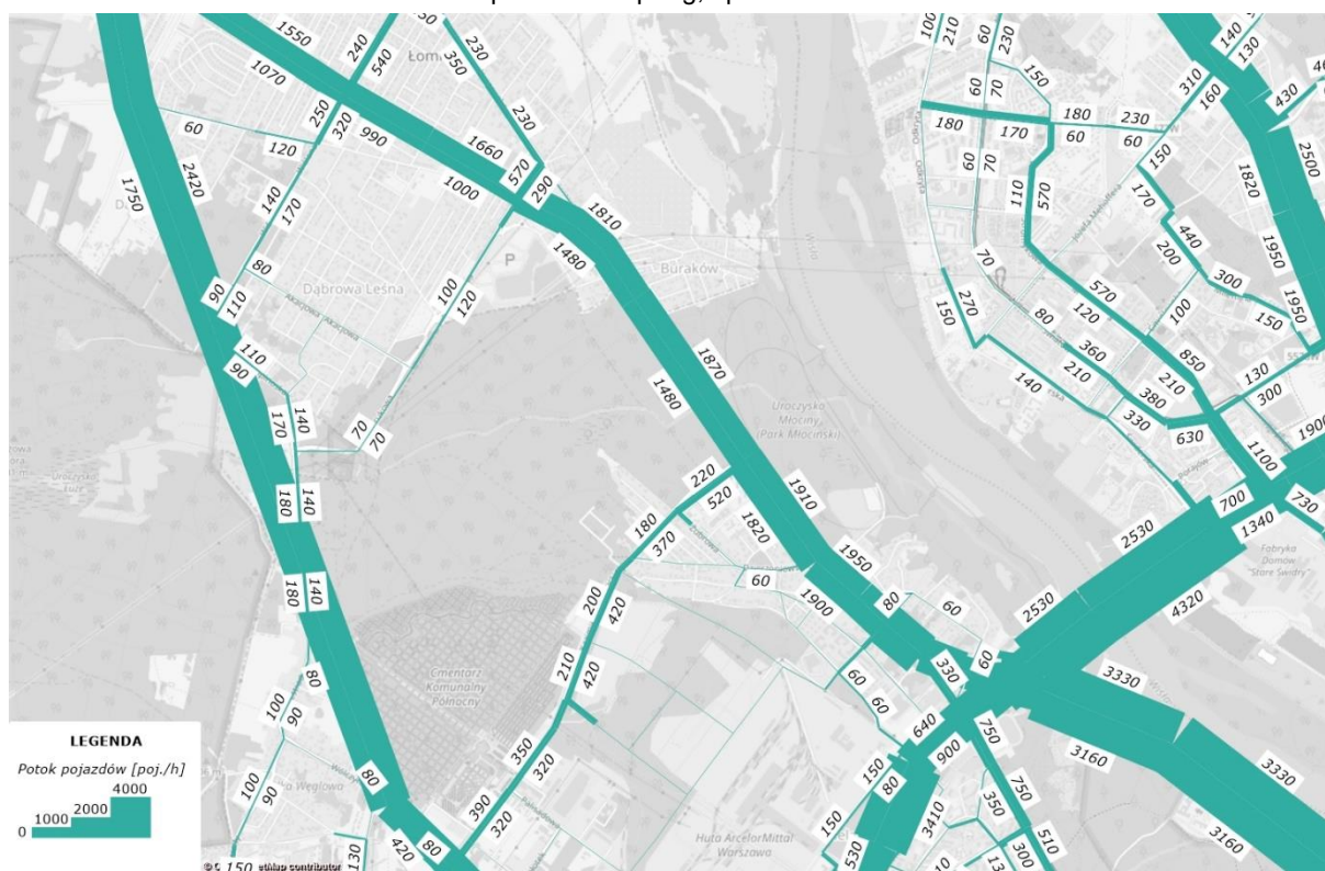
Rys. 6.36 Prognoza ruchu drogowego w szczycie popołudniowym w roku 2025 - warianty inwestycyjne WA i WB źródło: openstreetmap.org, opracowanie własne
