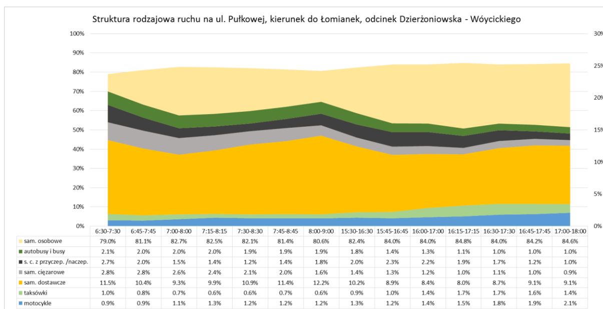
Rys. 4.21 Wyniki pomiarów ruchu, struktura rodzajowa ruchu na ul. Pułkowej, kierunek do Łomianek, odcinek Dzierżoniowska - Wóycickiego (źródło: opracowanie własne)
