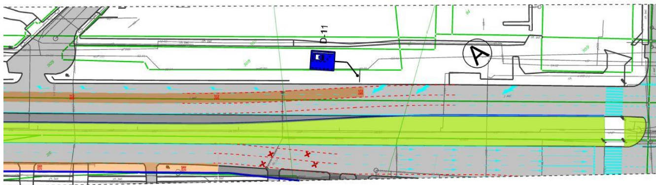
Rys. 5.17. Miejsce rozpoczęcia pasa autobusowego (na wylocie ze skrzyżowania z ul. Muzealną, w miejscu, gdzie kończy się pas włączeń) – wariant 1b, podwariant z poszerzeniem ul. Pułkowej z wykorzystaniem pasa dzielącego.
