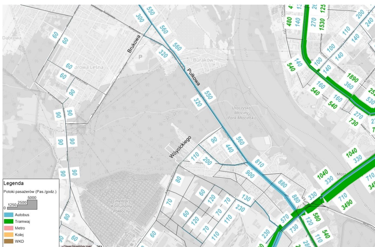
Rys. 6.32. Prognoza liczby pasażerów w szczycie popołudniowym w roku 2025 - wariant bezinwestycyjny W0 źródło:openstreetmap.org, opracowanie własne.
