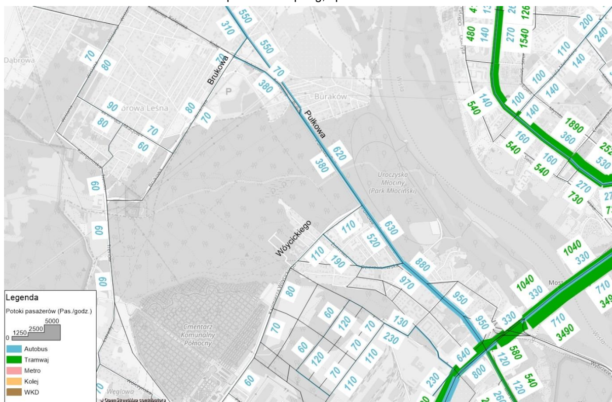
Rys. 6.34. Prognoza liczba pasażerów w szczycie popołudniowym w roku 2025 - wariant inwestycyjny WB źródło: openstreetmap.org, opracowanie własne
