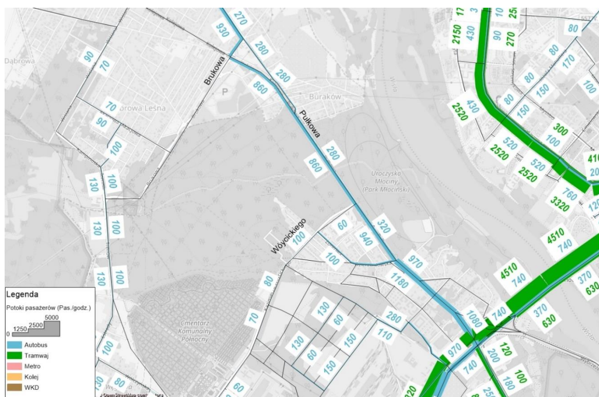
Rys. 6.28. Prognoza liczby pasażerów w szczyte poranne w roku 2025 – wariant bezinwestycyjny W0 źródło:openstreetmap.org, opracowanie własne
