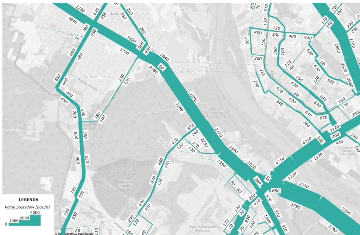
Rys. 6.21 Prognoza ruchu drogowego w szczycie porannym w roku 2020 - wariant bezinwestycyjny W0 źródło:openstreetmap.org, opracowanie własne
