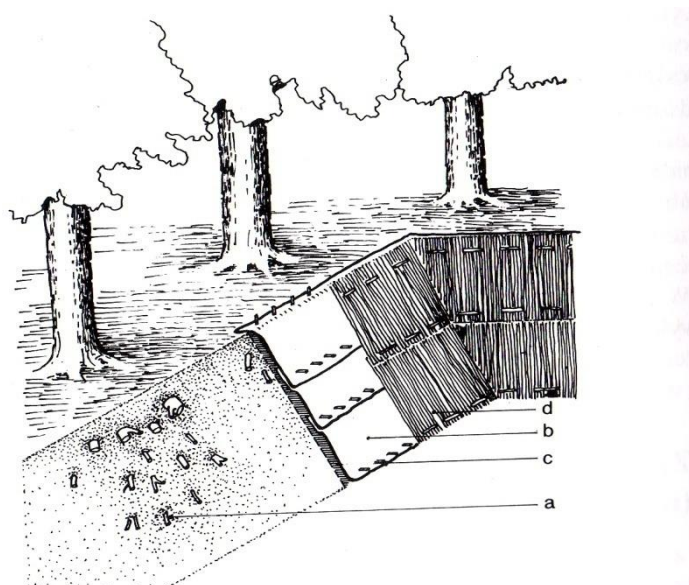
Rysunek 3 Zabezpieczanie korzeni w wykopie wg Chachulski Z. 2000 „Chirurgia i pielęgnacja drzew”: a) sposób przycięcia korzeni na krawędzi wykopu b) osłonięcie ściany wykopu warstwą torfu a następnie przykrycie folią lub jutą c) kołeczek mocujący osłonę do ziemi d) w przypadku wykonywania prac ziemnych w okresie mrozów należy dodatkowo użyć maty słomianej
