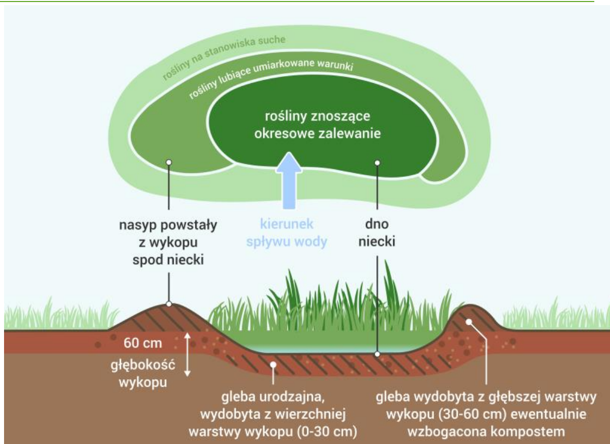
Rysunek 9 Schemat tworzenia infiltracyjnej niecki retencyjnej oraz jej budowy 22
