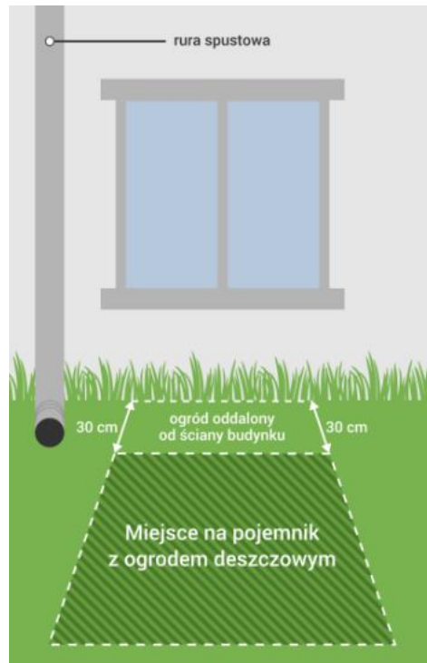
Rysunek 7 Schemat lokalizacji ogrodu deszczowego w pojemniku 20
