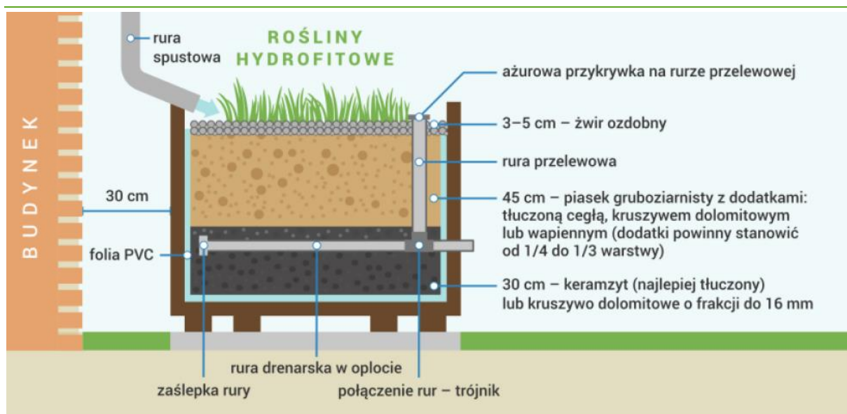
Rysunek 8 Schemat budowy ogrodu deszczowego w pojemniku 21
