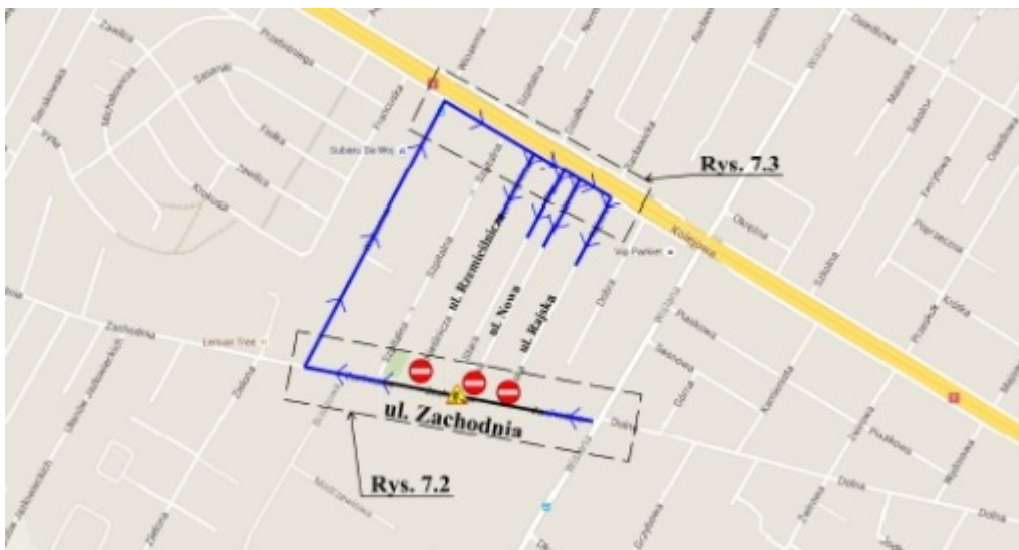
Etap III B - Przebudowa chodnika na odcinku od ul. Rzemieśniczej do ul. Zielonej (kliknij w obrazek, żeby powiększyć)
